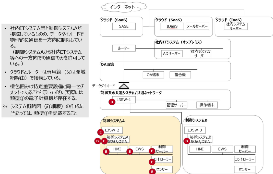
図8 制御系システムに常時リモートアクセスがあるパターン
